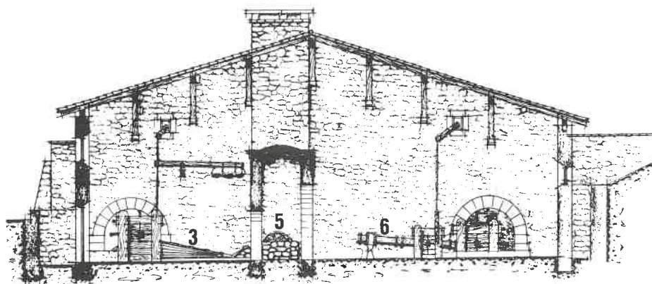
Mirandaola. Sección Oeste-Este.
