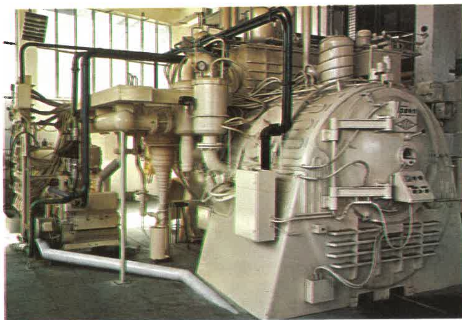
Horno de vacío COEL para tratamientos térmicos.
